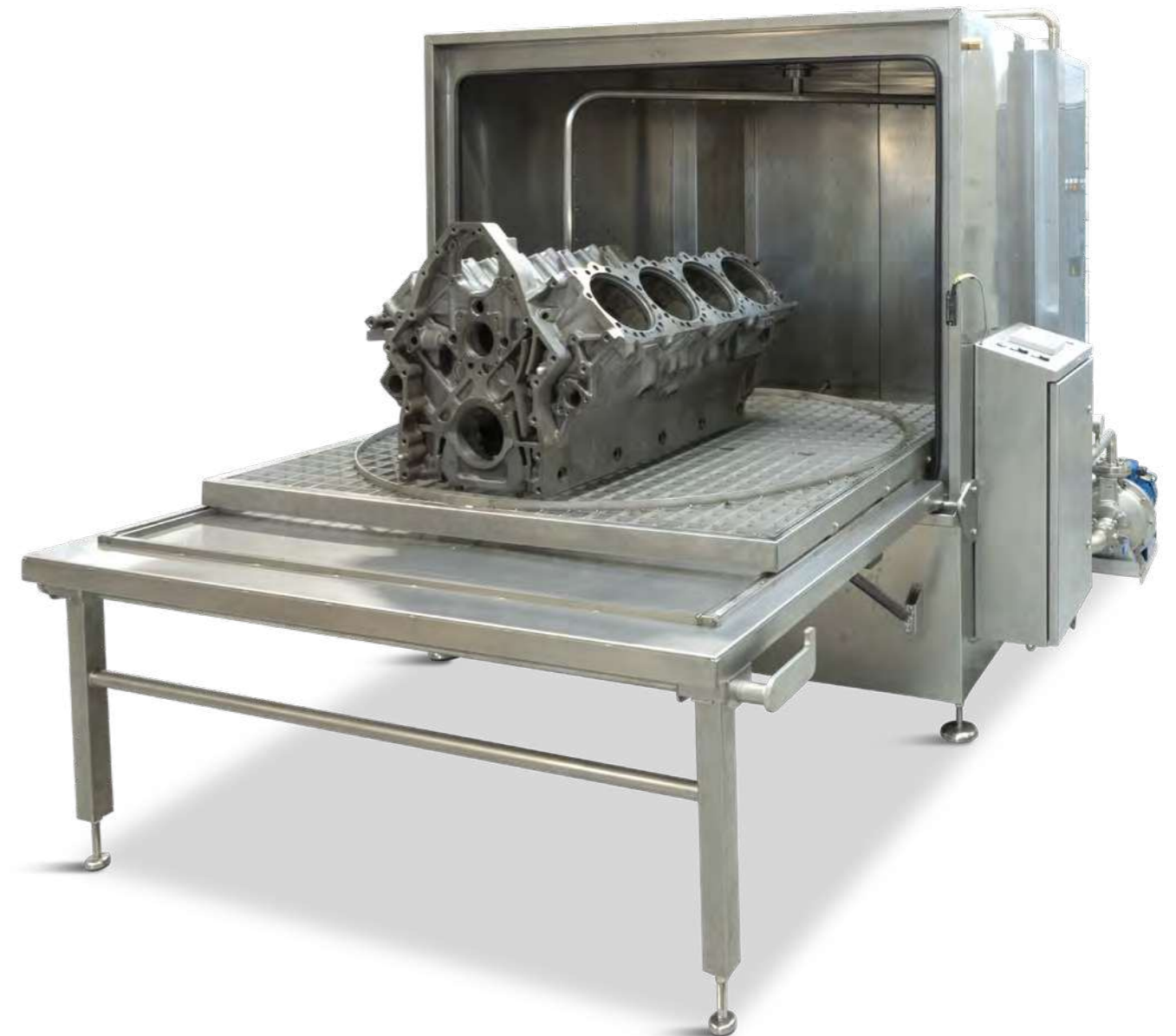
Zwei-Tanksystem
